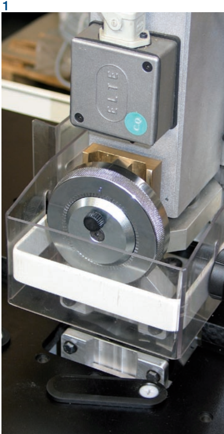
1 Gruppi refilatori ad alta frequenza con regolazione semplice ed immediata della asportazione tramite ghiera girevoli ad indicazione decimale (brevetto scm).
